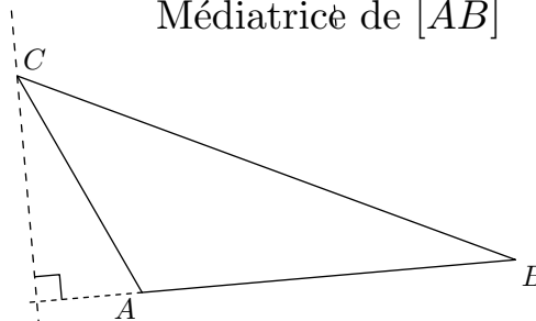
Hauteur issue de C
