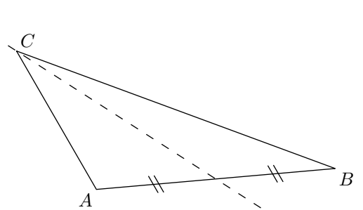
Médiane issue de C
