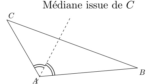
Bissectrice de l'angle \widehat{CAB}
