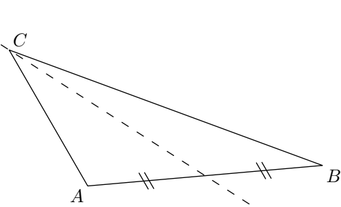
Médiane issue de C
