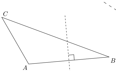
Médiatrice de [AB]
