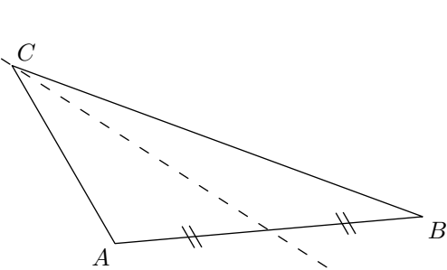
Médiane issue de C
