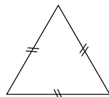
Triangle équilatéral
