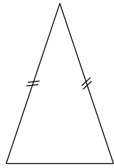
Triangle isocèle
