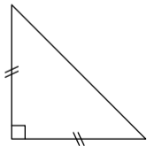
Triangle isocèle rectangle
